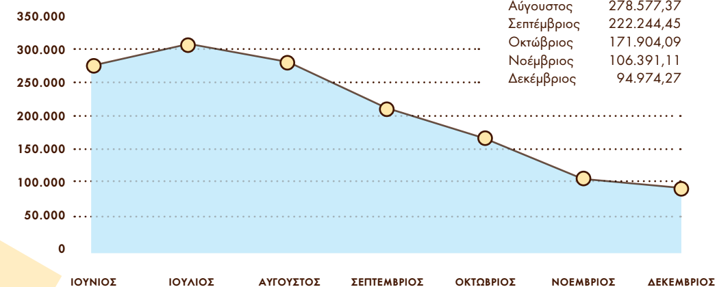
Ενέργεια από το στέγαστρο (kWhs)
